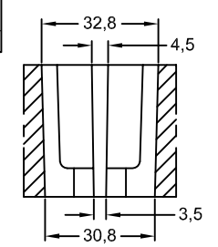
DOORSNEDE B-B
